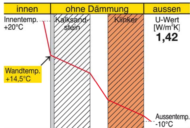
Temperaturverlauf eines ungedämmten Mauerwerks
