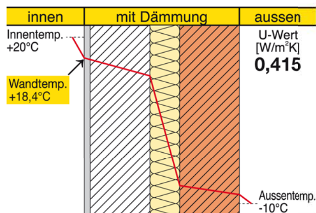
Temperaturverlauf eines mit DUROLAN gedämmten Mauerwerks bei einer typischen Außenwand eines Hauses der 60er/70er Jahre
